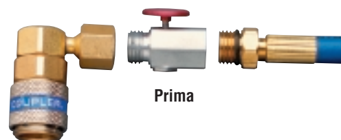
C52704 Raccordo per il lato a bassa pressione R-134a Purge-Mate con pulsante di disaerazione. Basta premere il pulsante per spurgare l'aria.
